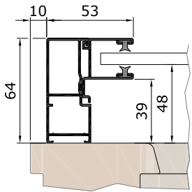
Führungsschiene KD53RA
