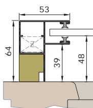
Thermisch getrennte Führungsschiene KD53VT
